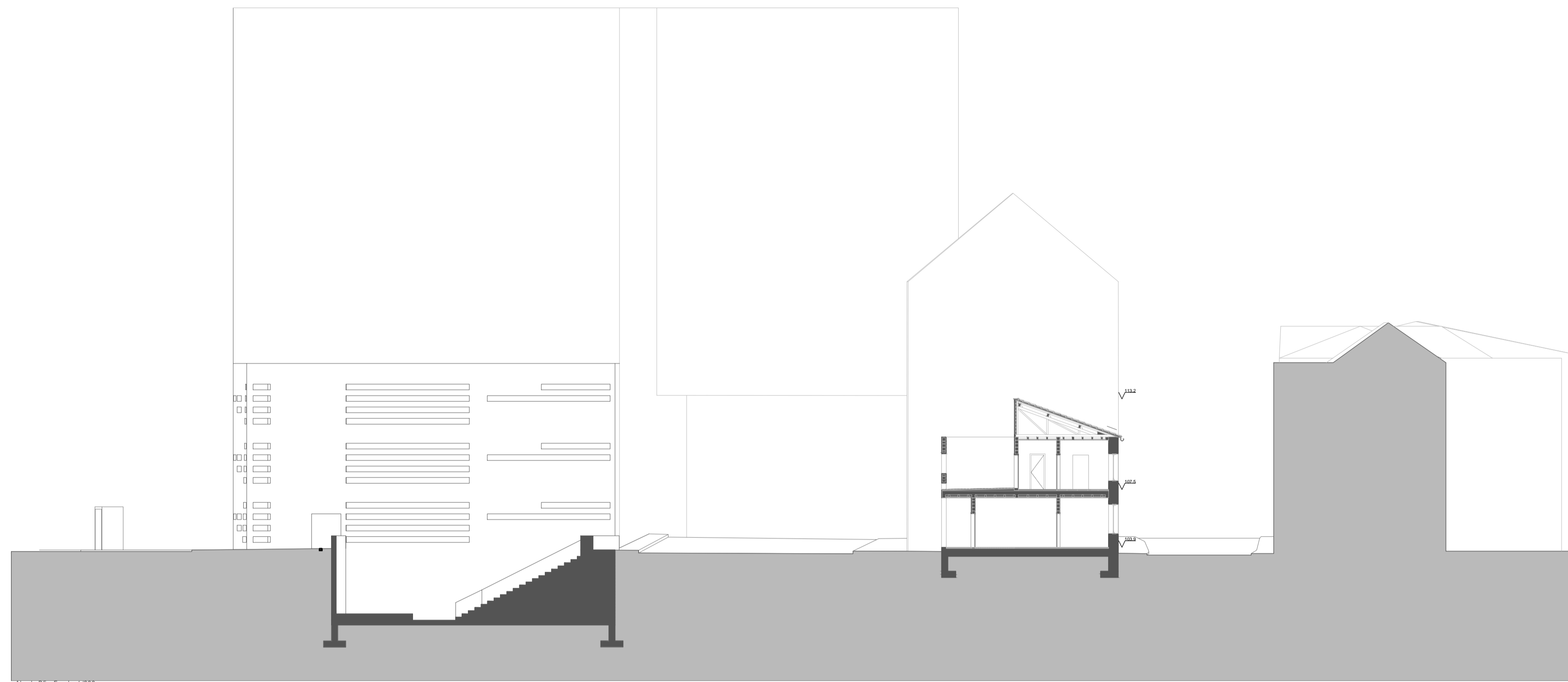
Algado B5 - Escala: 1/200
