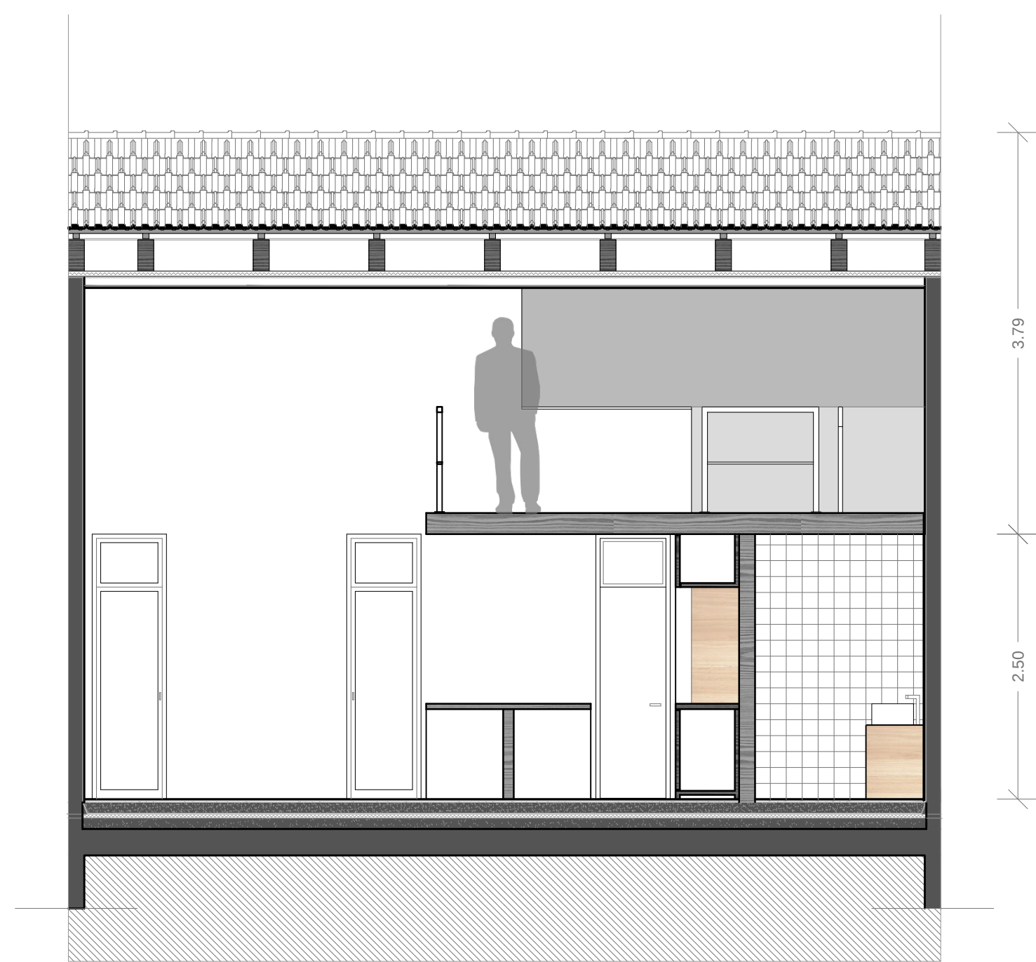
Corte C
