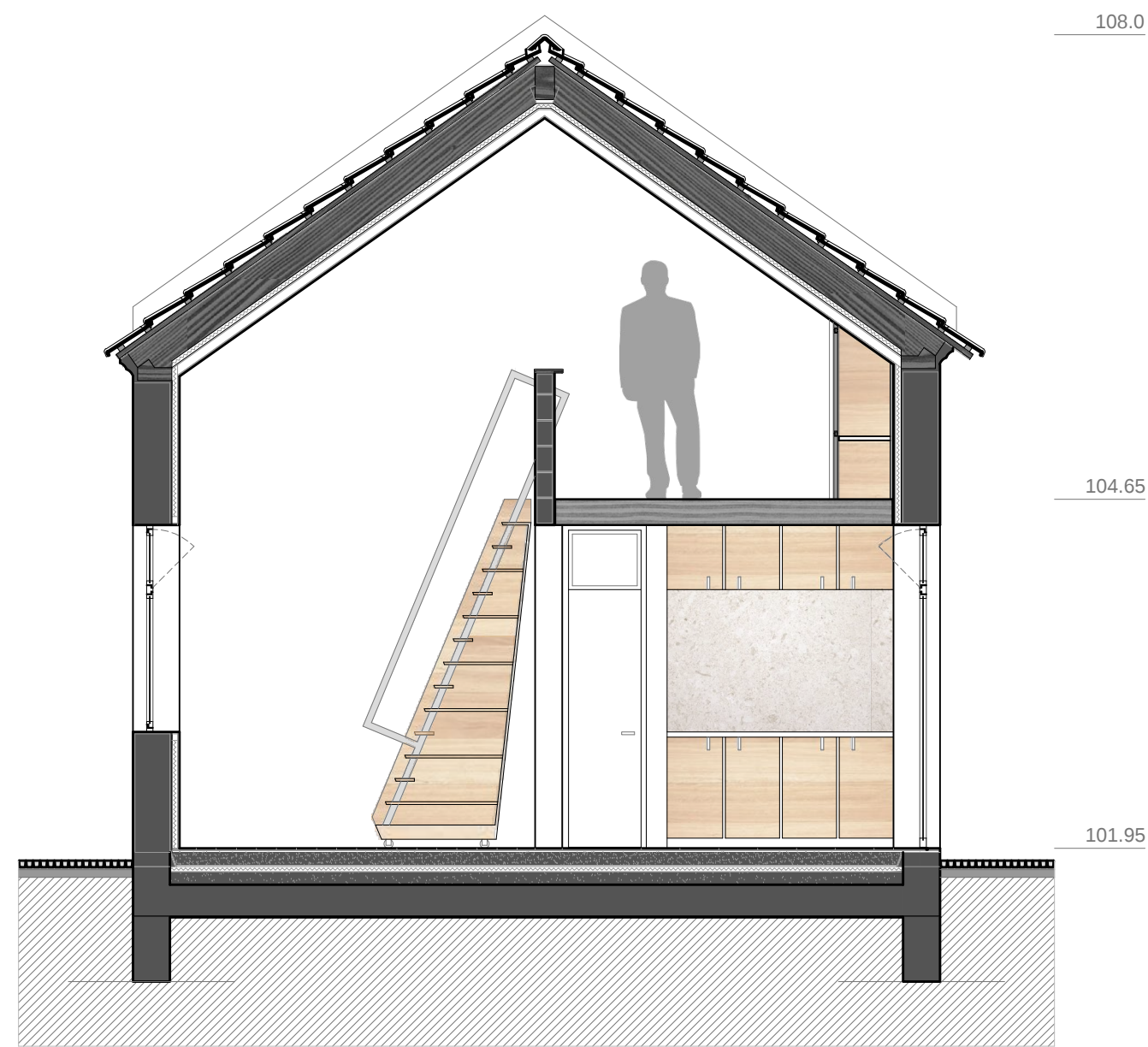
Corte B
