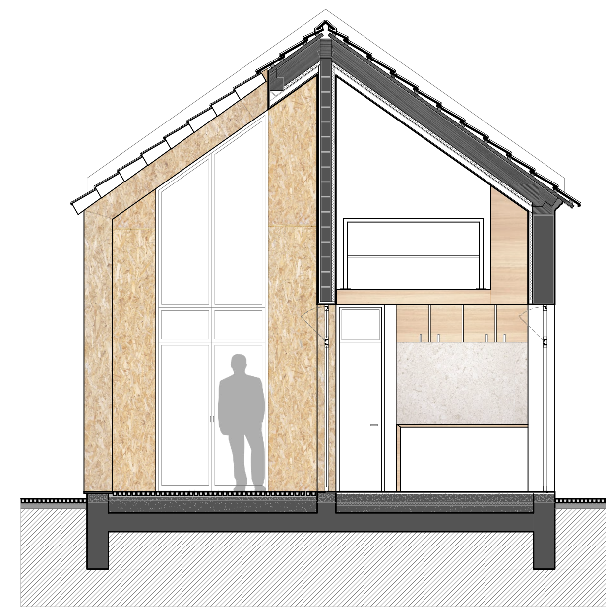
Corte A
