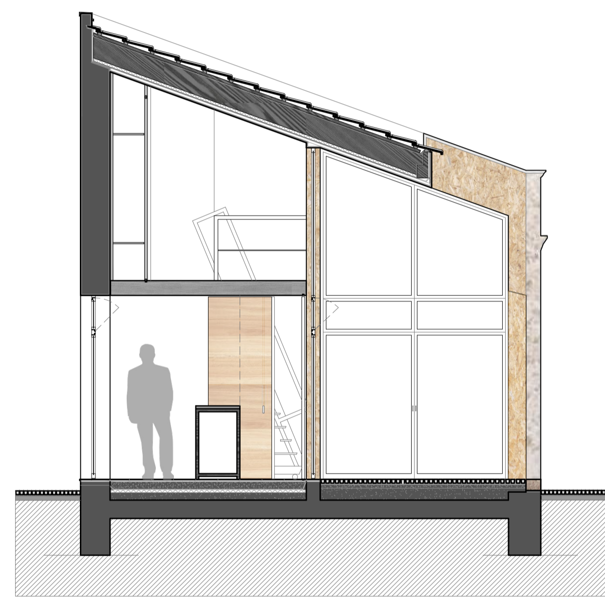
Corte A
