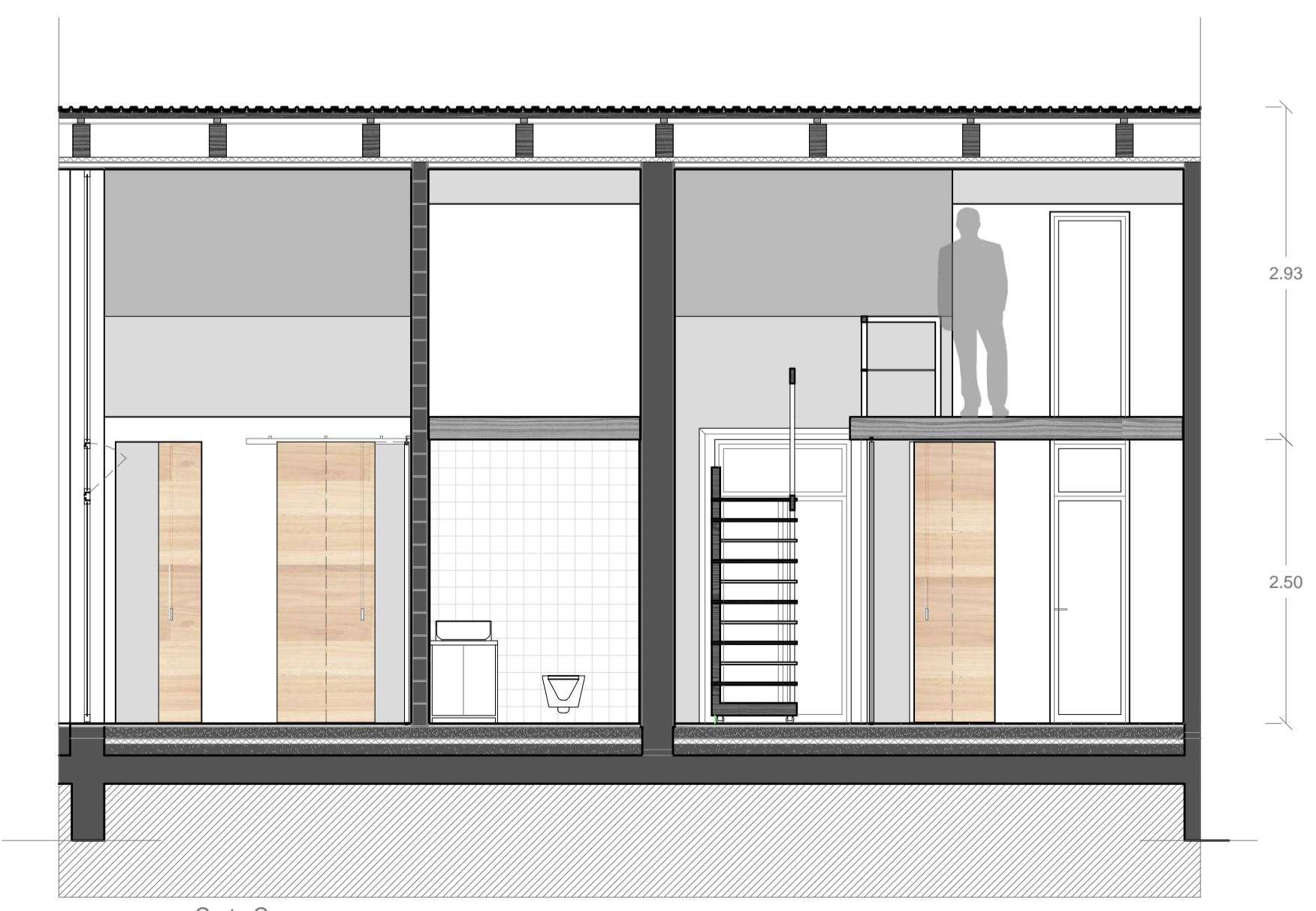
Corte C
