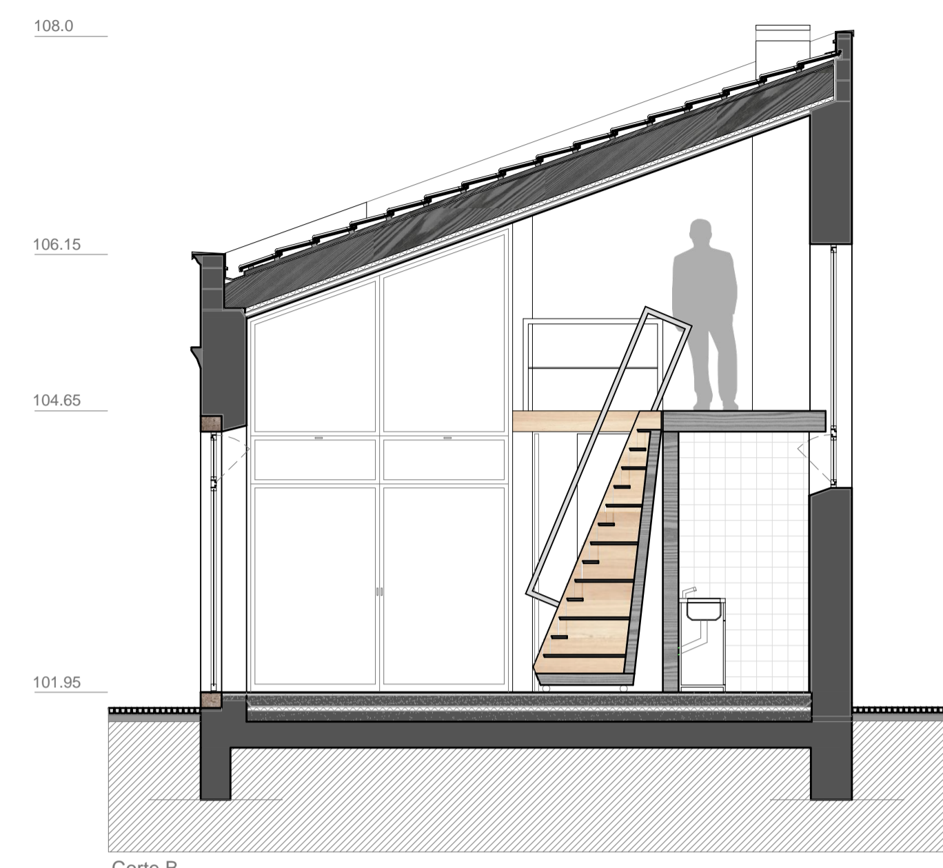
Corte B
