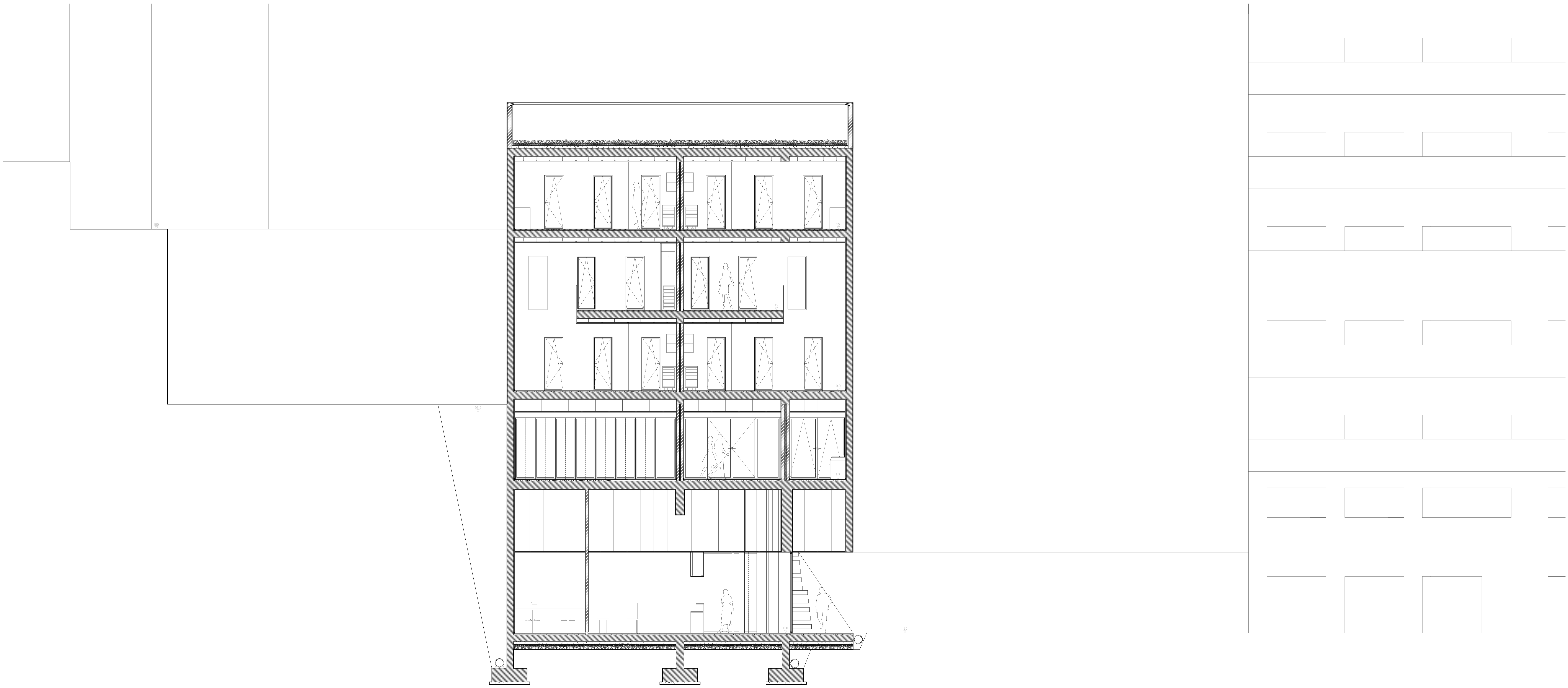
Corte D
