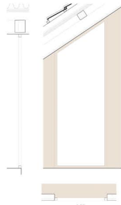
Ve03 tipo: construção: acabamento: vão de 1 folha fixa porta com caixilho de madeira com perfil de encaixe e vidro fixado madeira à vista
