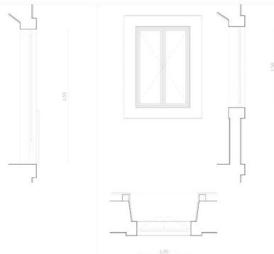
Ve03 tipo: construção: acabamento: vão de 2 folhas de batente porta com caixilho em madeira de perfil com encaixe e vidro fixado com brasa mate
