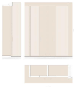
Ve04 tipo: construção: acabamento: vão de 1 folha de correr porta com perfil de madeira laminada colada cruzado à mão ou colado, madeira à vista
