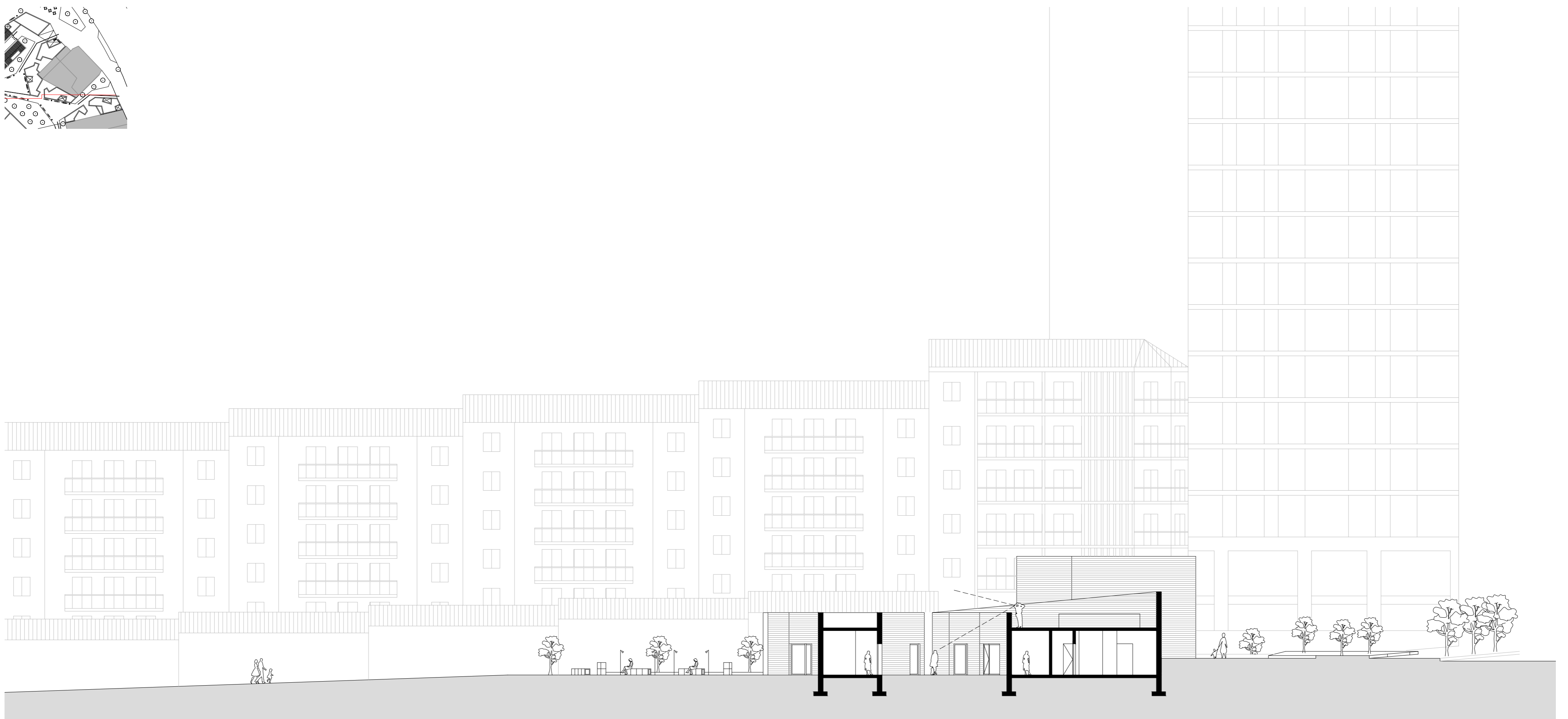
Corte d-4 (habitação nº1 e nº2)
