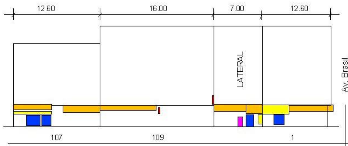
Figura 2.30 - Imagem gráfica da localização dos suportes nos edifícios nº107 a 1 (desenho Helena Almeida, 2013)
