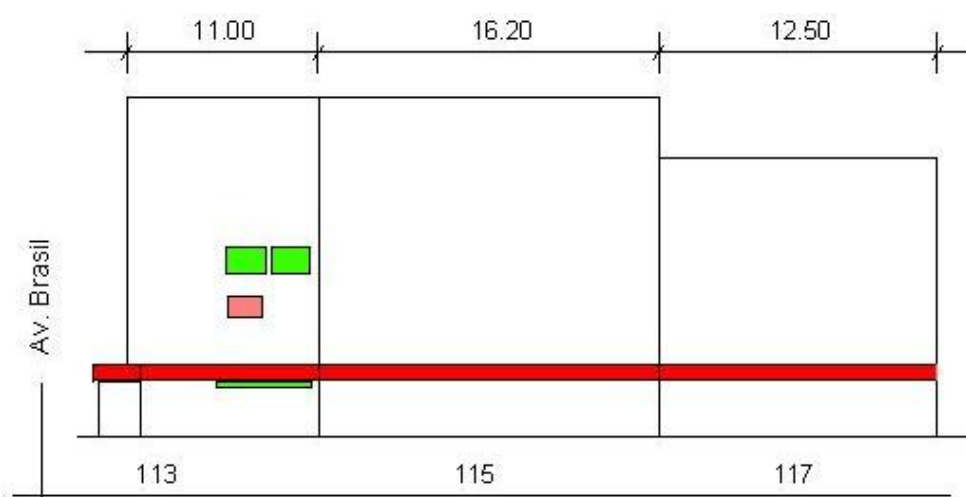
Figura 2.54 - Suportes publicitários nos edifícios de 113 a 117 - Situação Proposta (desenho Helena Almeida, 2013)
