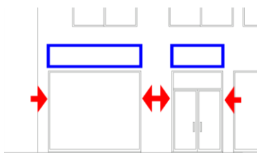
Figura 2.42 – Limites laterais para a colocação de anúncios (desenho Helena Almeida, 2013)
