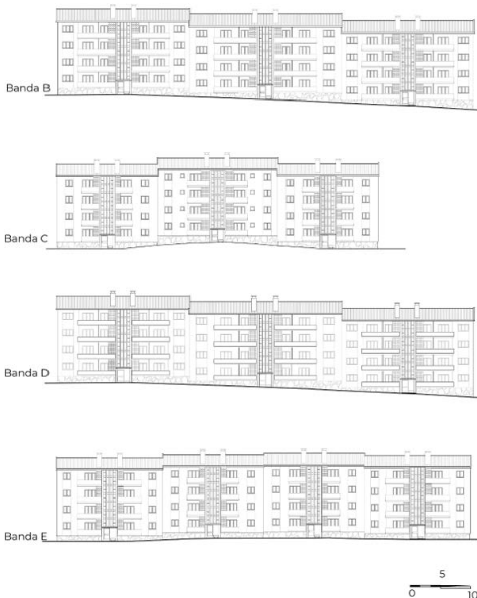
Figura 6. Alçados
