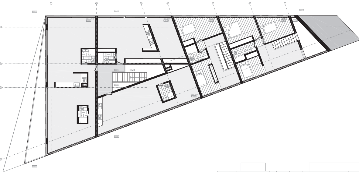
Piso 2 1_100
