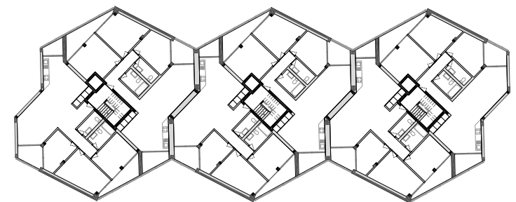
Planta do andar tipo proposta 0 5m 1m
