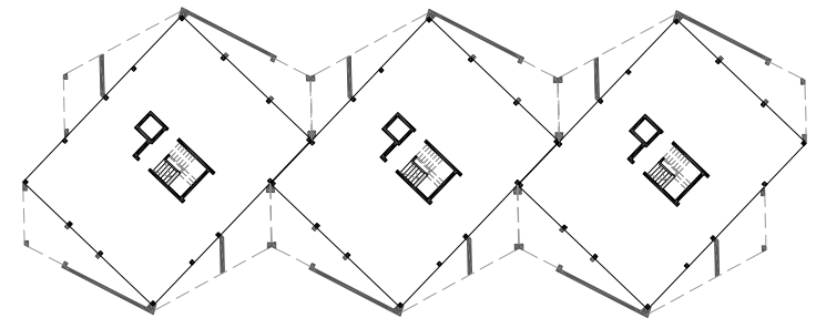
Estrutura existente e proposta
