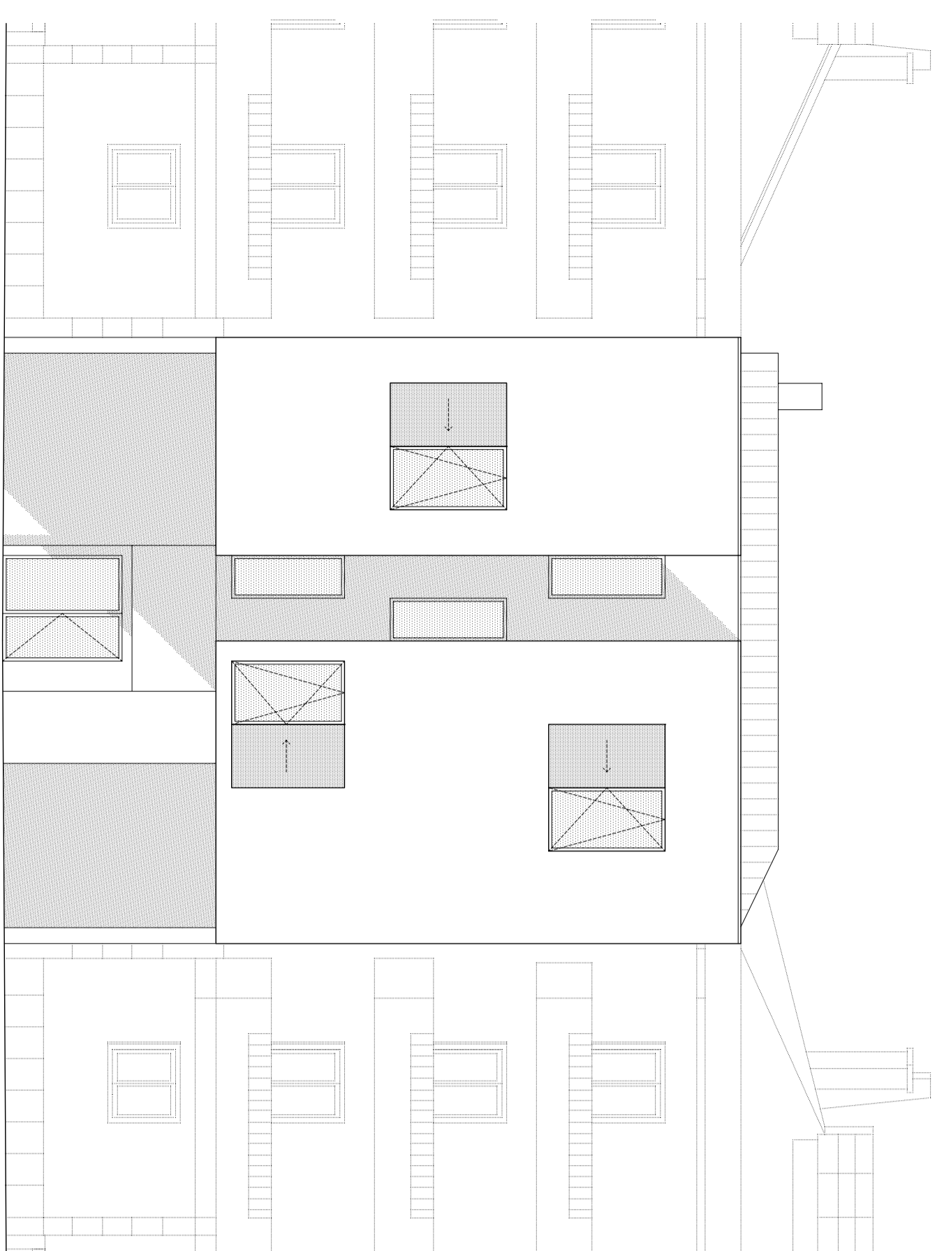
Alçado Norte escala 1/100
