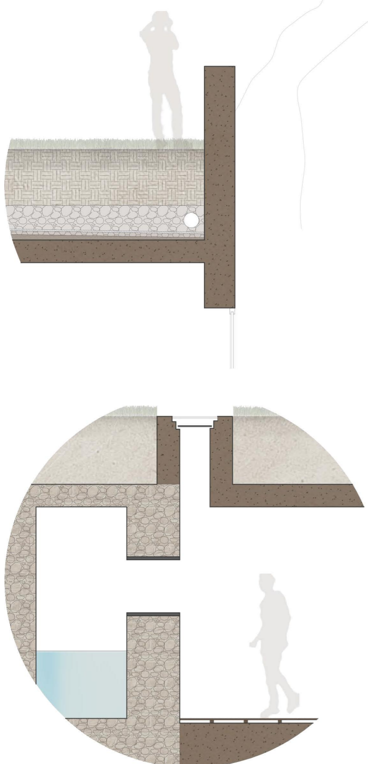
Promenor construtivo de abertura para luz
