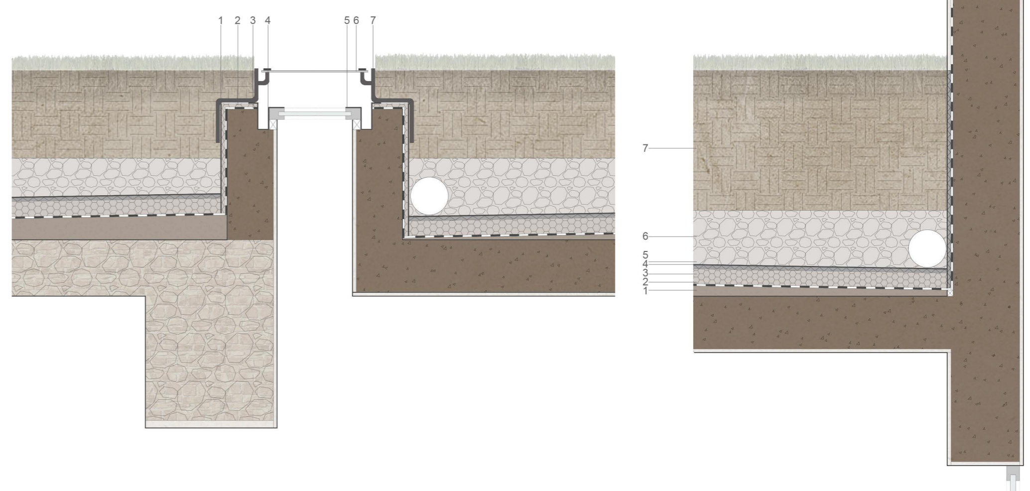
Promenor construtivo da cobertura ajardinada
