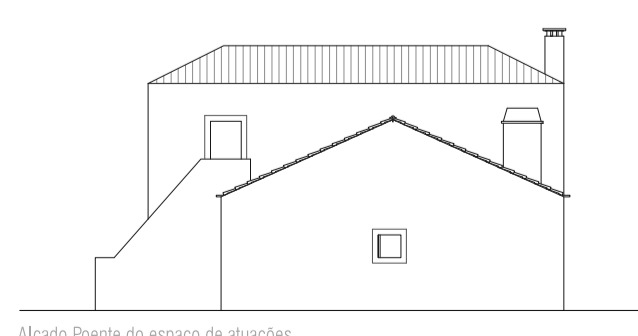
Alçado Poente do espaço de atuações
