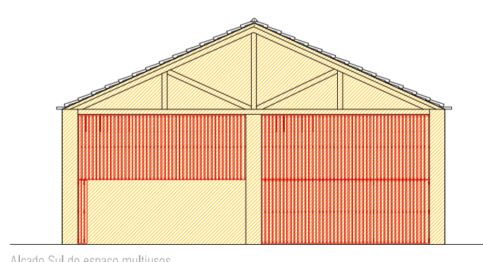
Alçado Sul do espaço multissos
