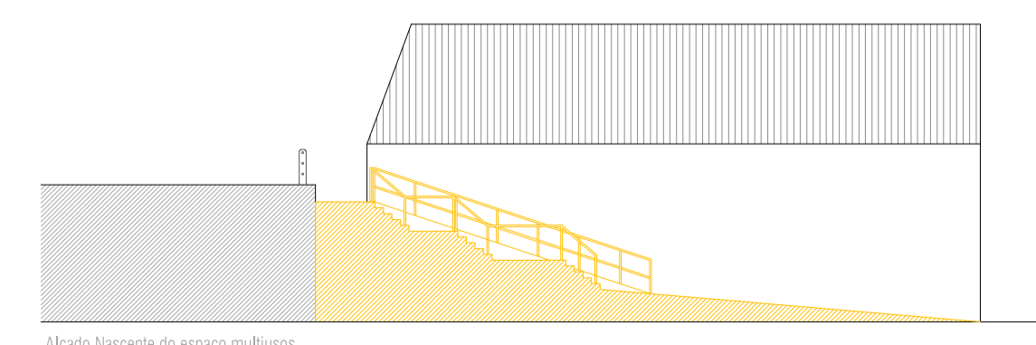
Alçado Nascente do espaço multissos
