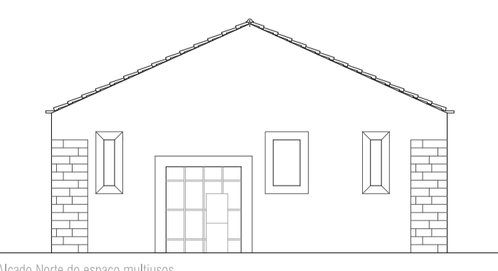
Alçado Norte do espaço multissos
