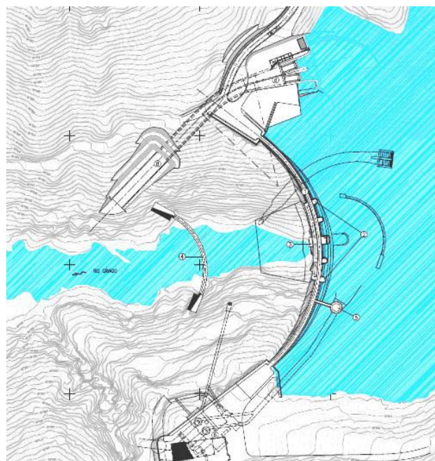
Figura 3.2 - Vista em planta da barragem de Salomonde e da intervenção realizada – DCC (LNEC, 2012).
