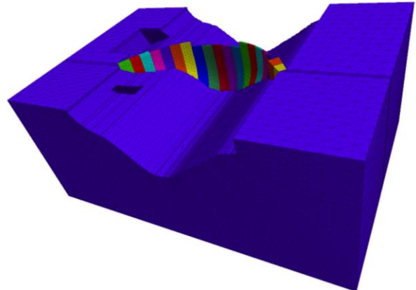
Figura 4.1 - Vista do modelo numérico da barragem e maciço de fundação.
