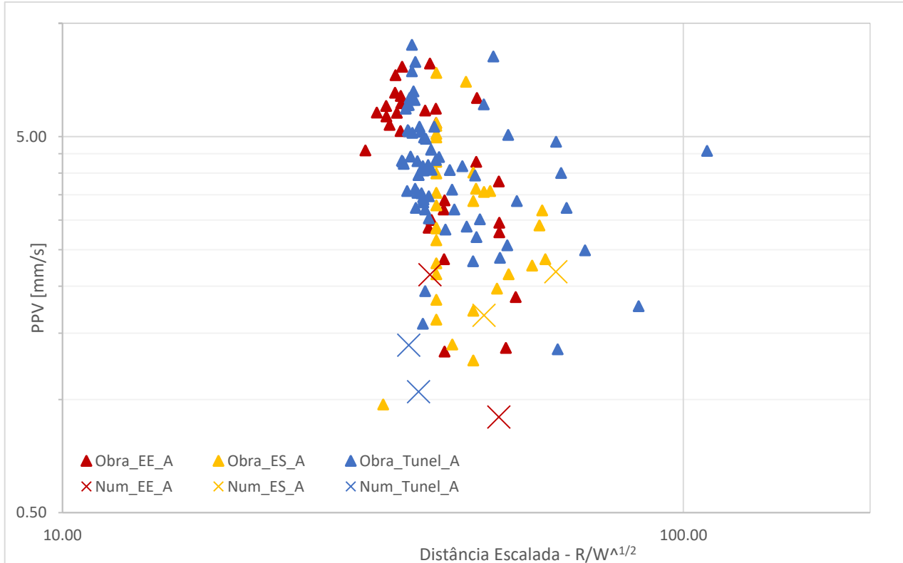
Figura 5.5 - Comparação dos resultados no ponto de controle A, correspondente ao coroamento, entre a simulação de pegas no modelo numérico com as medições em obra.
