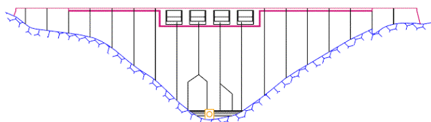
Figura 3.1 – Alçado da barragem de Salomonde.
