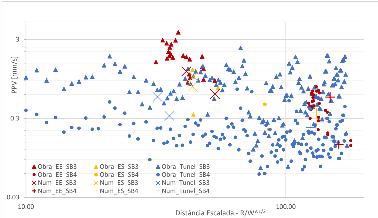
Figura 5.4 - Comparação dos resultados nos pontos de controle SB3 e SB4, correspondentes à fundação, entre a simulação de pegas no modelo numérico com as medições em obra.
