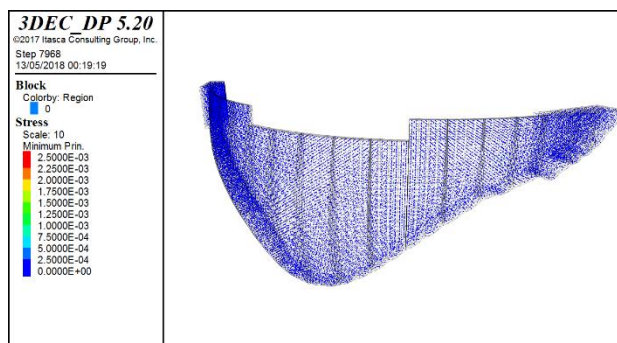
Figura 5.3 - Vista de jusante da barragem com representação das tensões provocadas por uma pega na estrutura de saída (ES).
