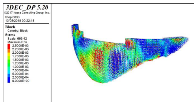
Figura 5.1 - Vista de montante da barragem com representação das tensões provocadas por uma pega na estrutura de entrada (EE).
