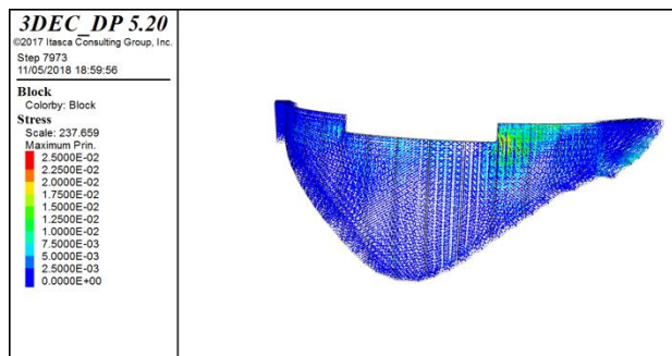
Figura 5.2 – Vista de jusante da barragem com representação das tensões provocadas por uma pega na estrutura do túnel (Túnel).
