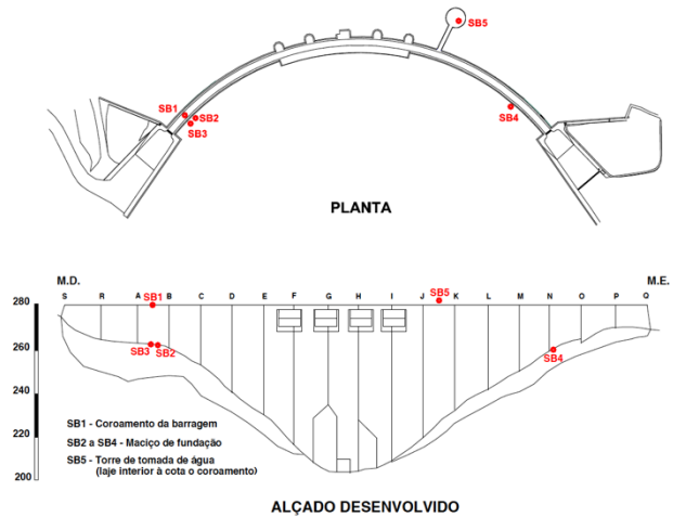
Figura 3.4 - Plano de colocação dos sismómetros na barragem (LNEC, 2012).
