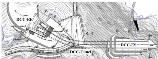
Figura 3.3 - Localização das três frentes de trabalho na execução do desmonte de rocha com uso de explosivos do DCC (LNEC, 2012).
