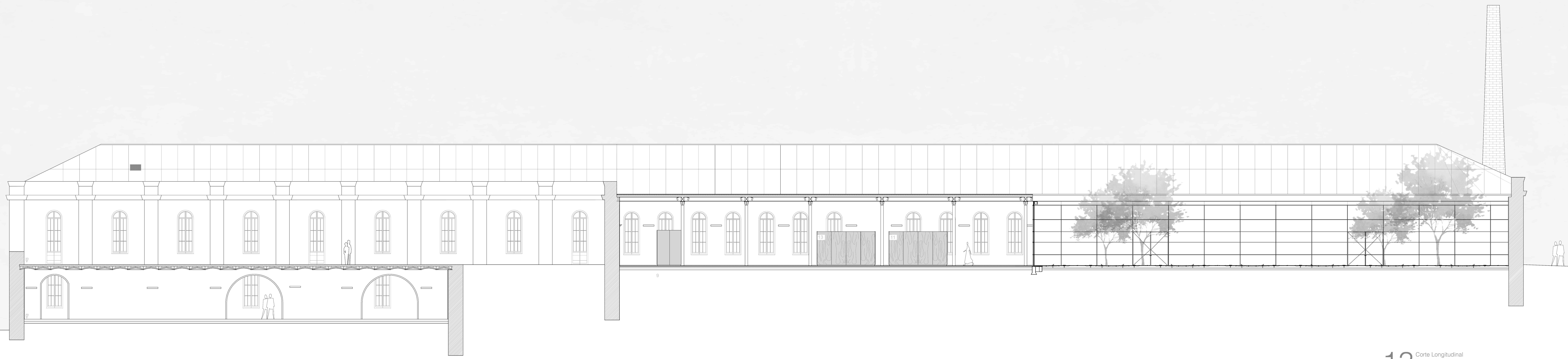
13 Corte Longitudinal Escala 1:100 Joana Alves | nº 61201 | Projecto Final de Arquitectura | Prof. Pedro Pinto
