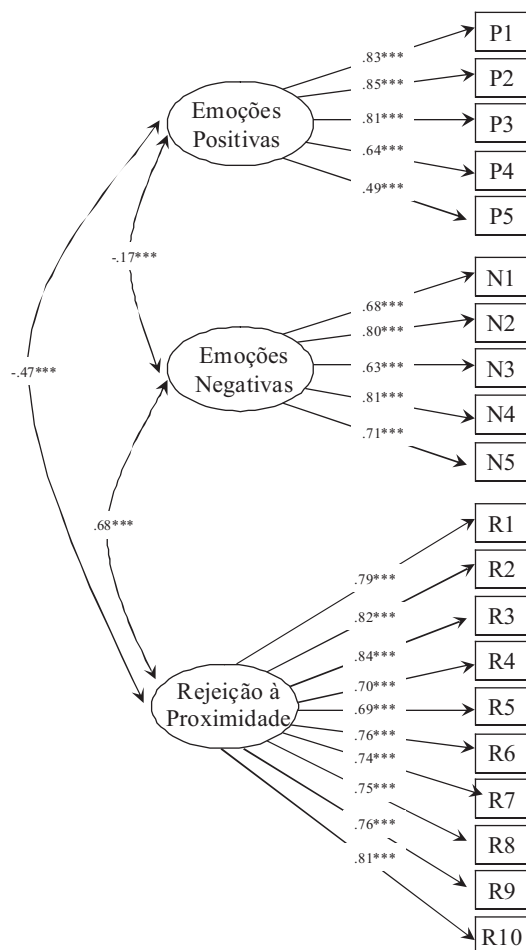
Figura 2. Análise factorial confirmatória das medidas de Preconceito contra os Homossexuais
