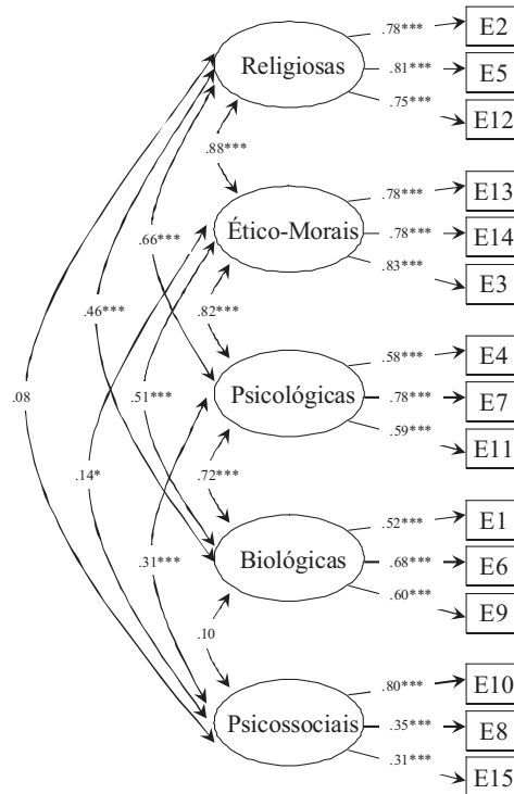
Figura 1. Análise factorial confirmatória da Escala de crenças sobre a natureza da homossexualidade
