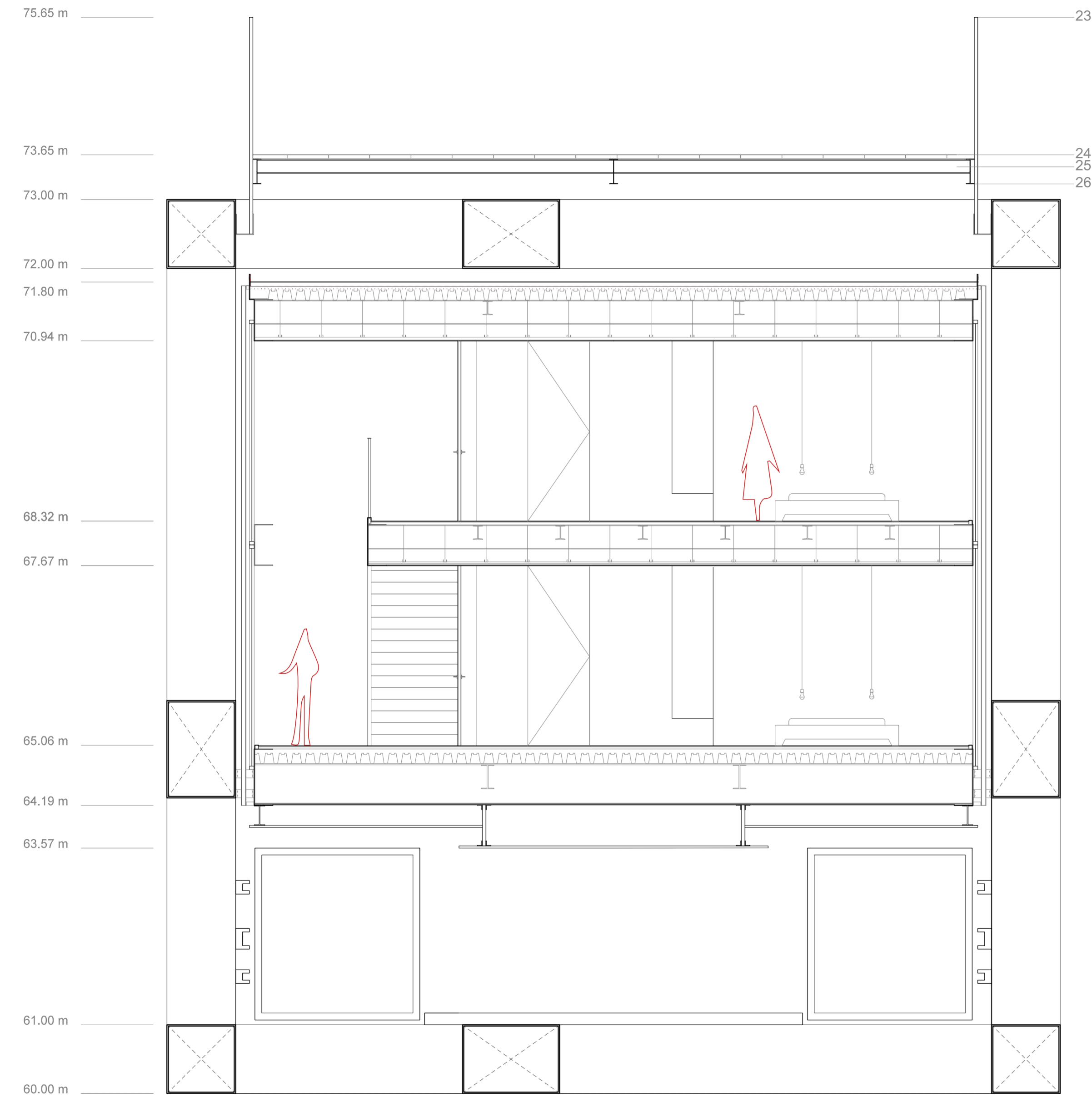
Corte transversal
