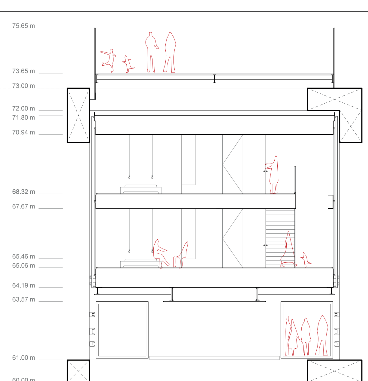
Corte MM'
