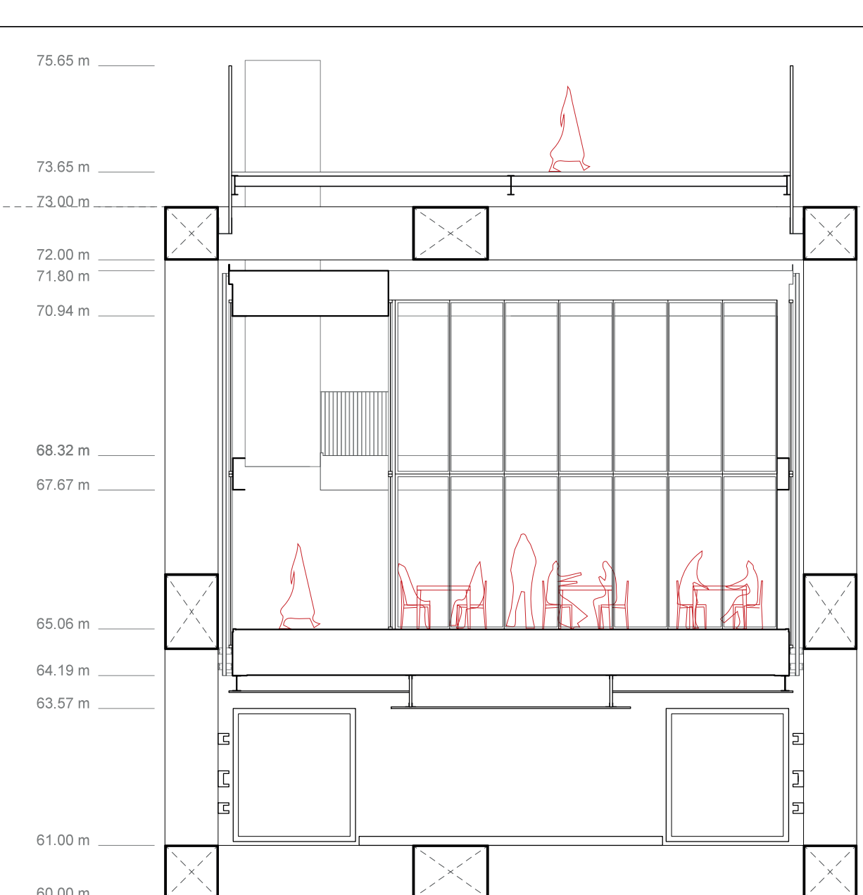
Corte PP'
