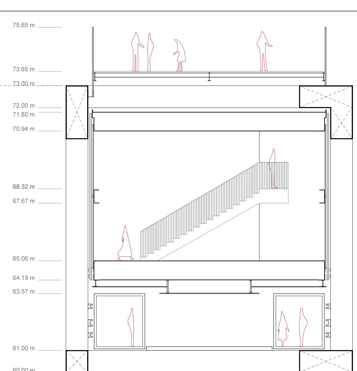
Corte NN
