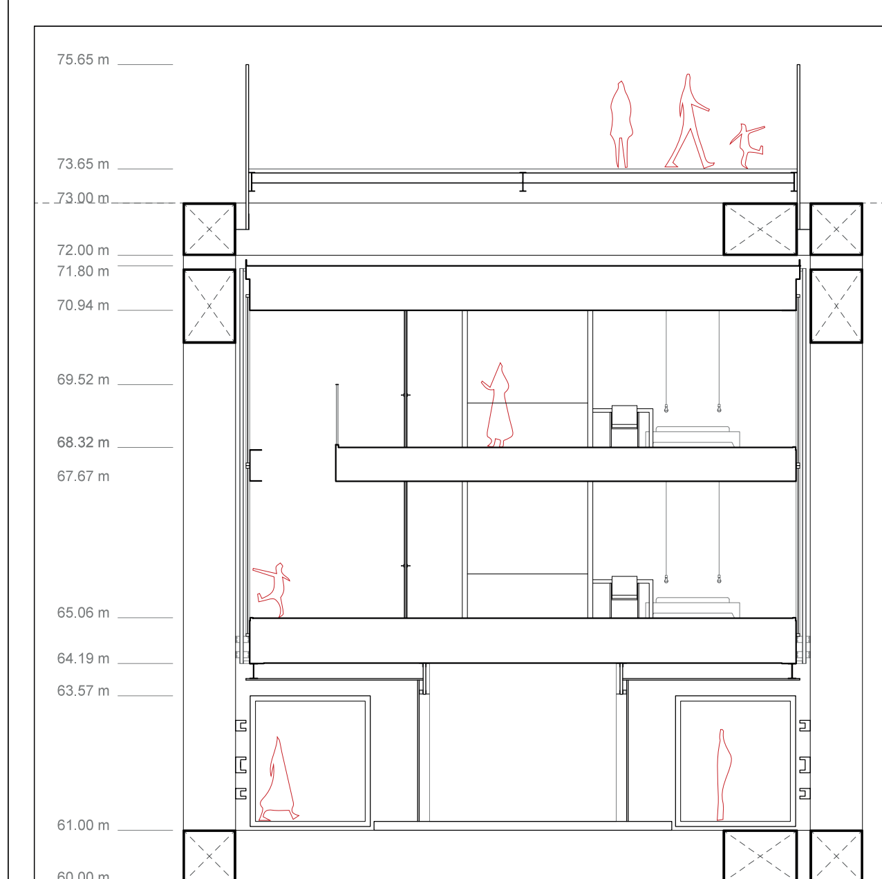
Corte KK'
