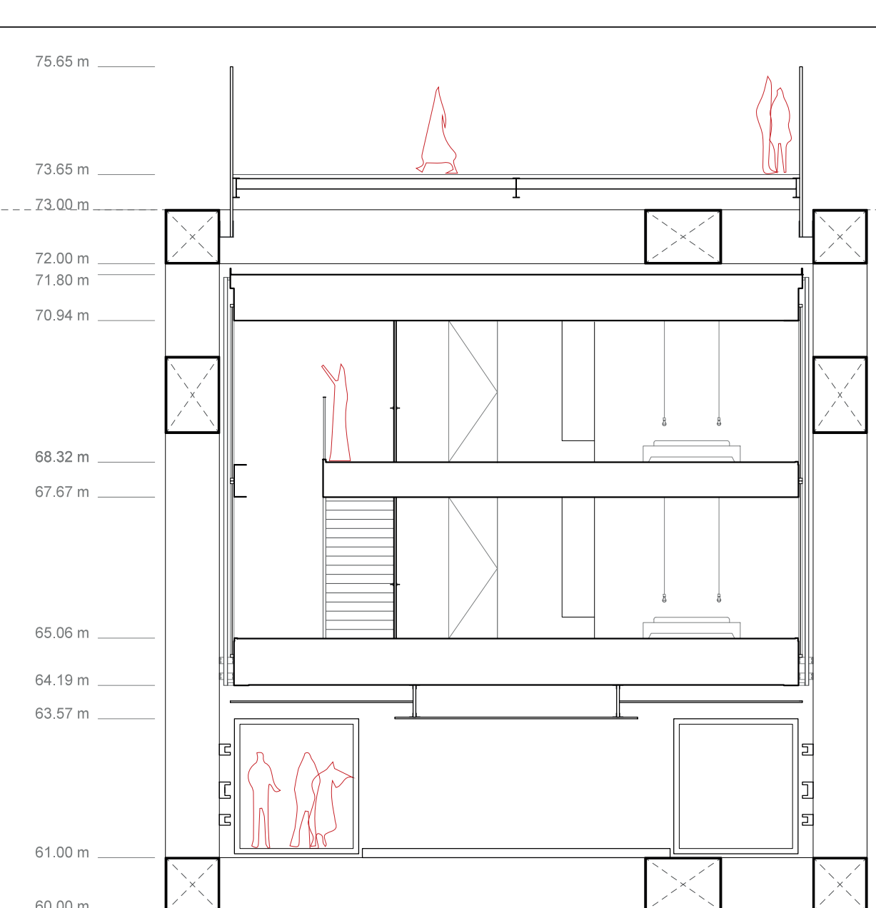
Corte OO'
