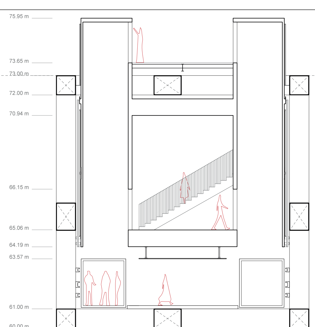
Corte LL'
